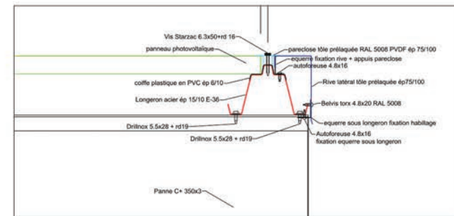
Coupe F-F
